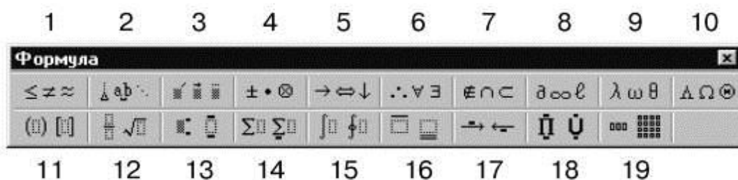
Рис. 3.1. Панель EquationEditor
